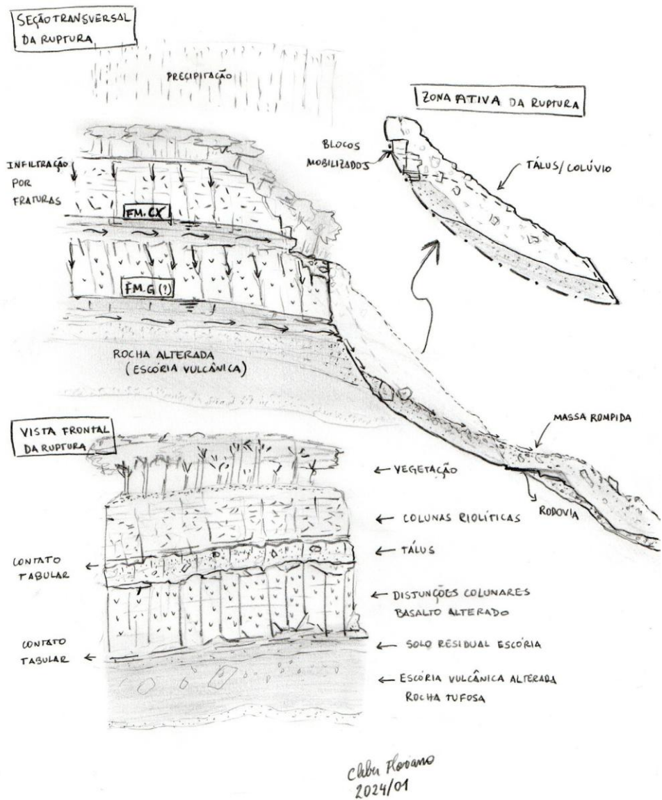
Figura 1 – Croqui demonstrando as principais feições geológicas basálticas e a relação com o mecanismo de ruptura em encostas. Bacia do Rio das Antas, estrada vicinal próxima a BR-470, município de Bento Gonçalves, região serrana da Formação Serra Geral, RS. Legenda e croqui (2024): Cleber Souza Floriano.
