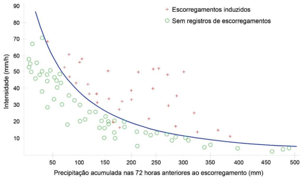
Figura 2 – Correlação entre chuva e escorregamentos induzidos. Serra do Mar, Cubatão, SP. Fonte: Tatizana et al., 1987, apud Cunha et al., 2022.
