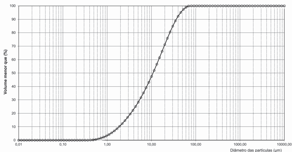
Figura 9. Curva Granulometrica dos sedimentos marginais do rio Amazonas, na comunidade São Braz. Fonte: Serviço Geológico do Brasil, Laboratório de Análises Mineraias - LAMIN Manaus.
