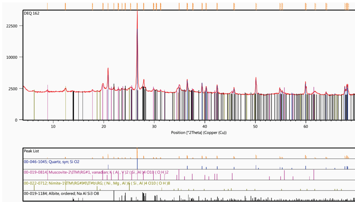
Figura 10. Perfil da difração raio - X da amostra coletada na margem direita do rio Amazonas - Comunidade São Braz. Fonte: Serviço Geológico do Brasil, Laboratório de Análises Mineraias - LAMIN Manaus.
