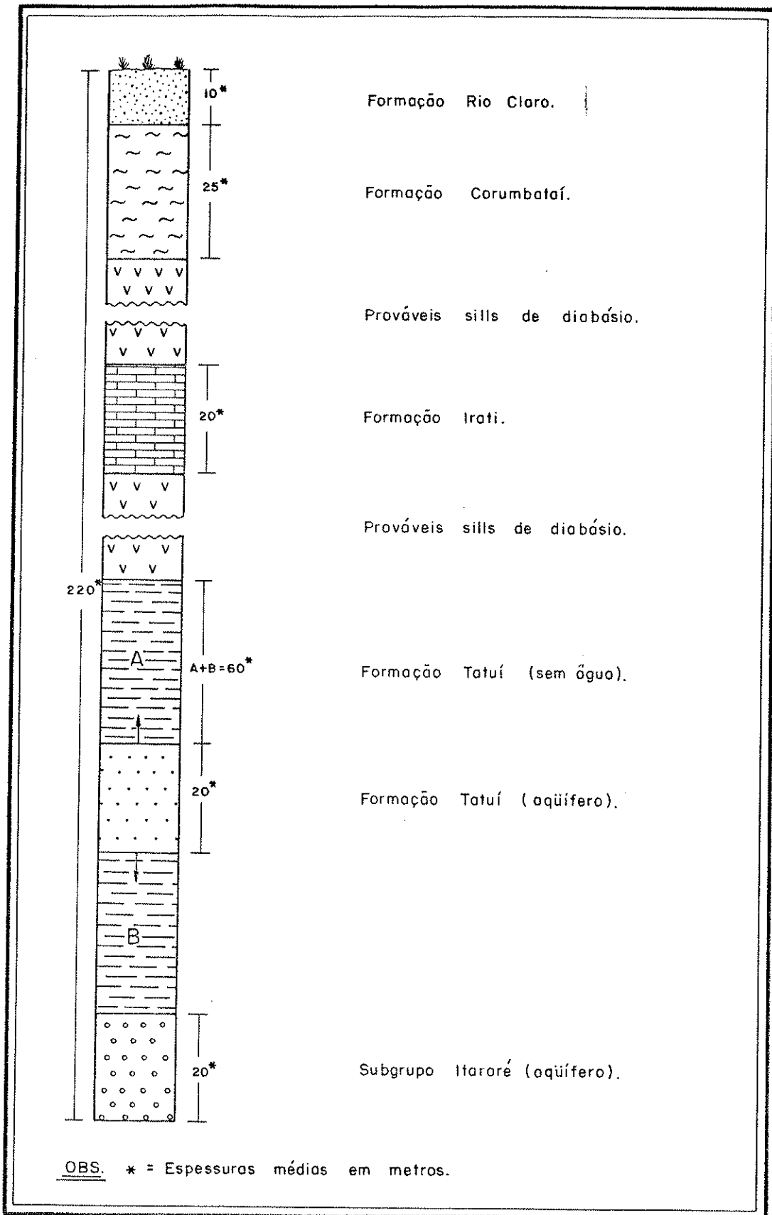
FIGURA 24: REPRESENTAÇÃO ESQUEMÁTICA DA ESTRATIGRAFIA NA ÁREA PESQUISADA PARA FINS HIDROGEOLOGÍCOS
