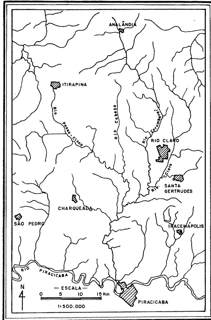
FIGURA 12: SISTEMA HIDROGRÁFICO DA REGIÃO DE RIO CLARO
