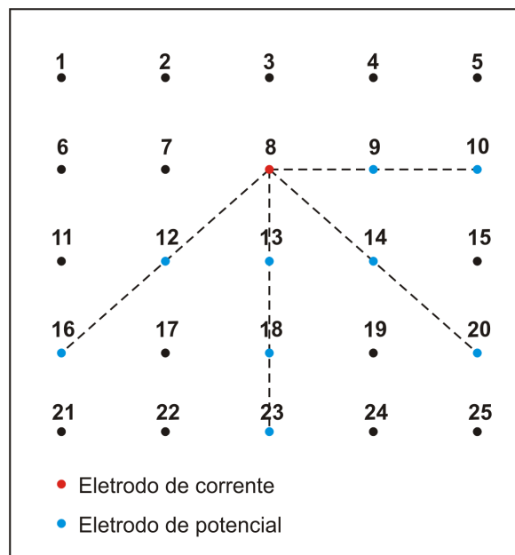
Figura 4.9 – Posição dos eletrodos de potencial correspondentes a um único eletrodo de corrente no arranjo 3D diagonal cruzado (modificado de LOKE e BARKER, op. cit.).
