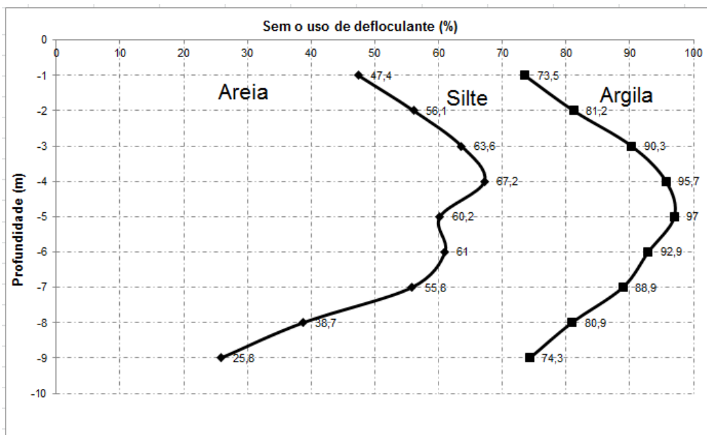
Figura 5.3. Variações das frações granulométricas sem o uso de defloculante do perfil com a profundidade.
