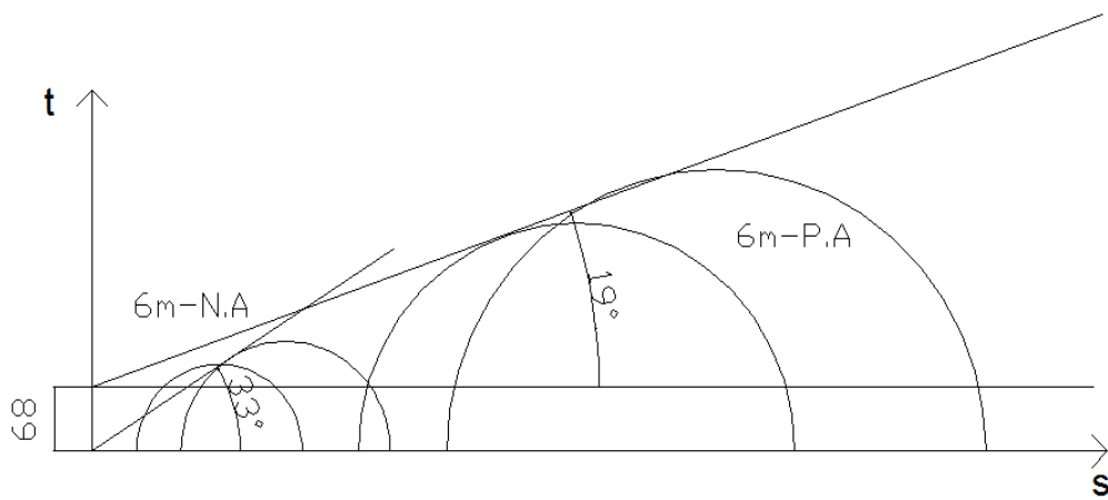
Figura II6- Envoltórias de resistência totais para o sexto metro.
