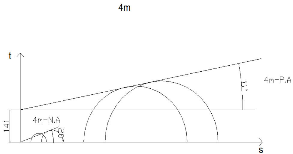
Figura II4- Envoltórias de resistência totais para o quarto metro.
