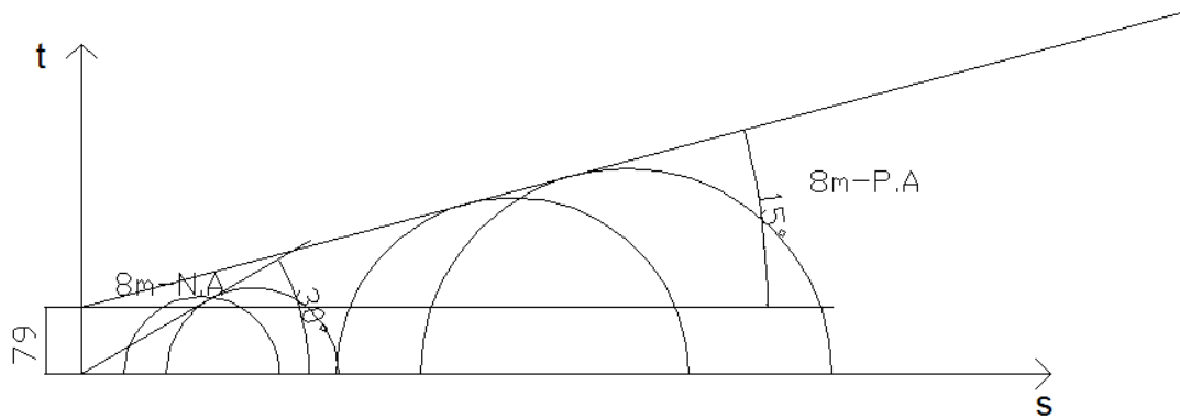
Figura II8- Envoltórias de resistência totais para o oitavo metro.
