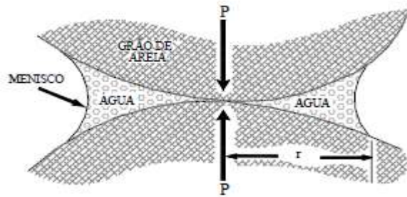
Figura 2.9. Arranjo estrutural devido à capilaridade (Dudley, 1970).
