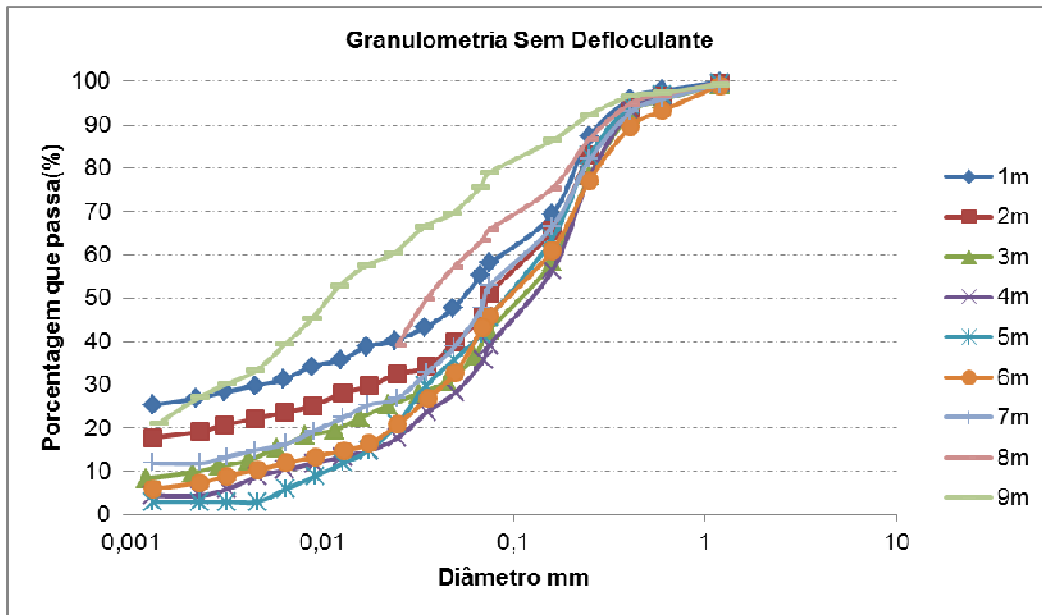
Figura 5.2. Curvas Granulométricas obtidas sem o uso de defloculante.
