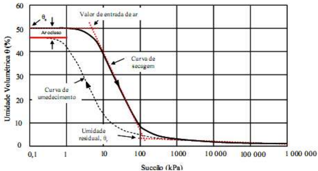
Figura 2.4 – Curva de retenção típica para um solo siltoso. (Fredlund e Xing, 1994).
