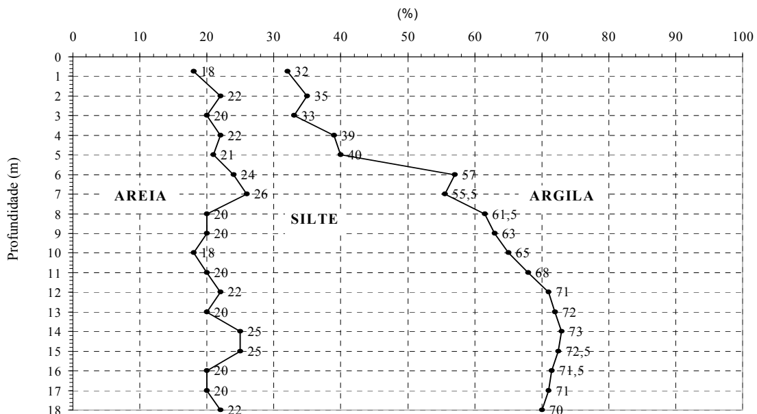
Figura 6.1 Variações das frações granulométricas do perfil com a profundidade do campo experimental da FEAGRI
