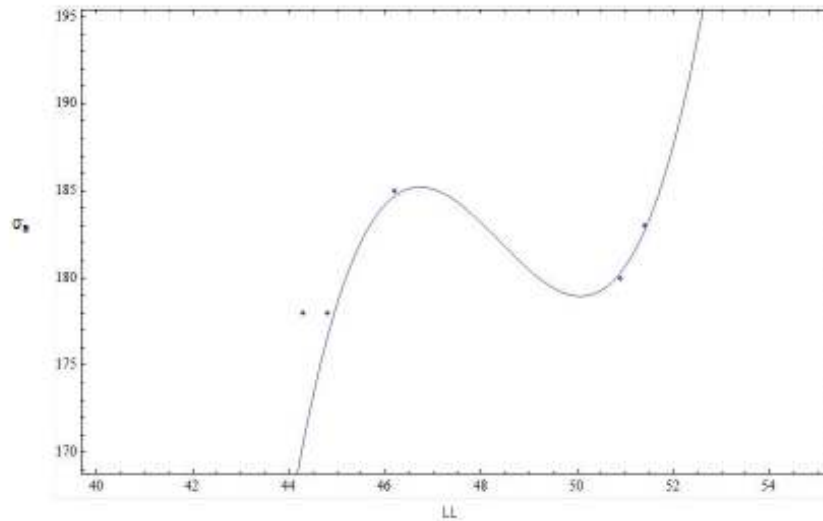
Figura 7.11 Modelo cúbico para correlação \sigma_a = f(LL)
