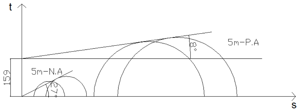
Figura II5- Envoltórias de resistência totais para o quinto metro.
