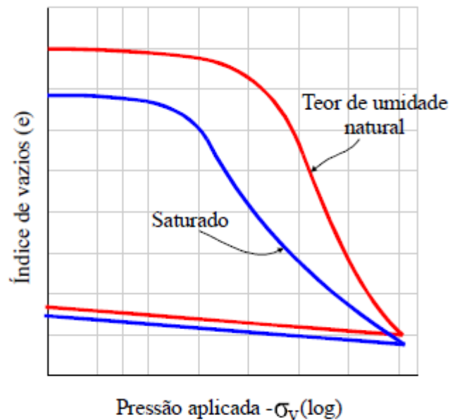
Figura 2.18. Curva e versus Log \sigma_v do ensaio edométrico duplo (Jennings e Knight, 1957).
