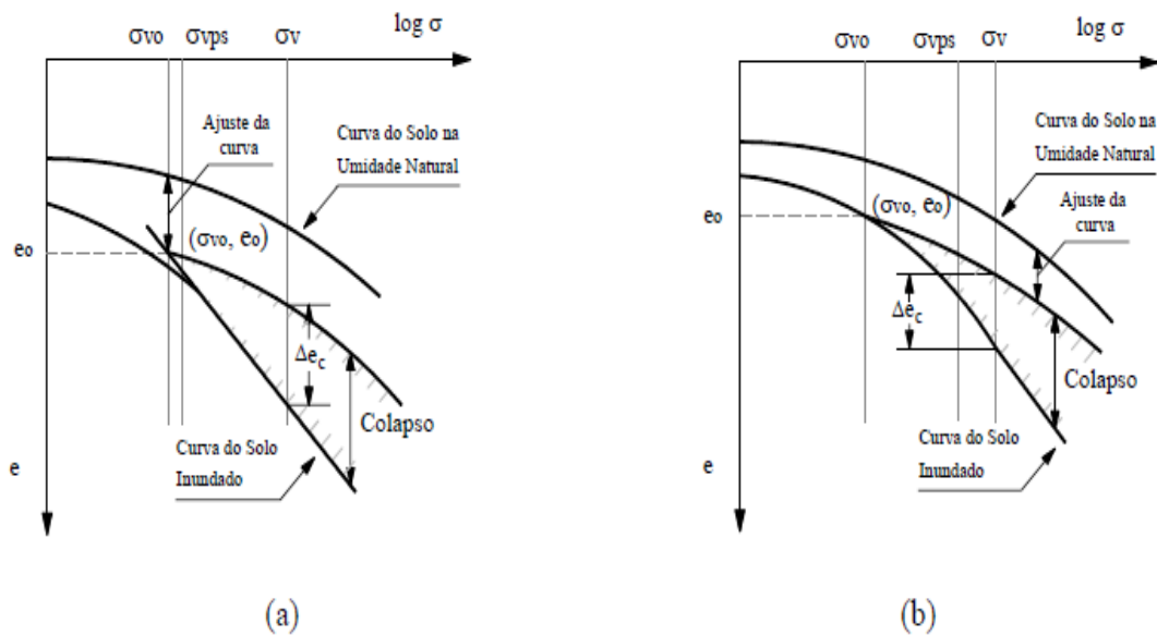
Figura 2.20 Ensaio duplo de adensamento (Jennings e Knight, 1957).
