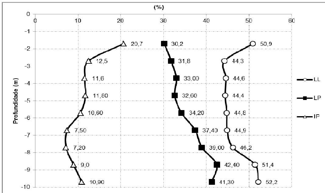
Figura 6.4 Variações dos limites de Atterberg em função da profundidade do campo experimental da FEC.
