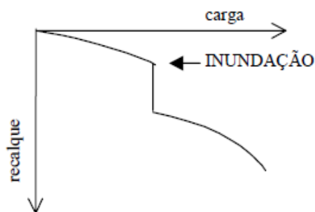
Figura 2.16. Conceito básico de recalque adicional devido ao colapso da estrutura do solo (Jennings e Knight, 1975).
