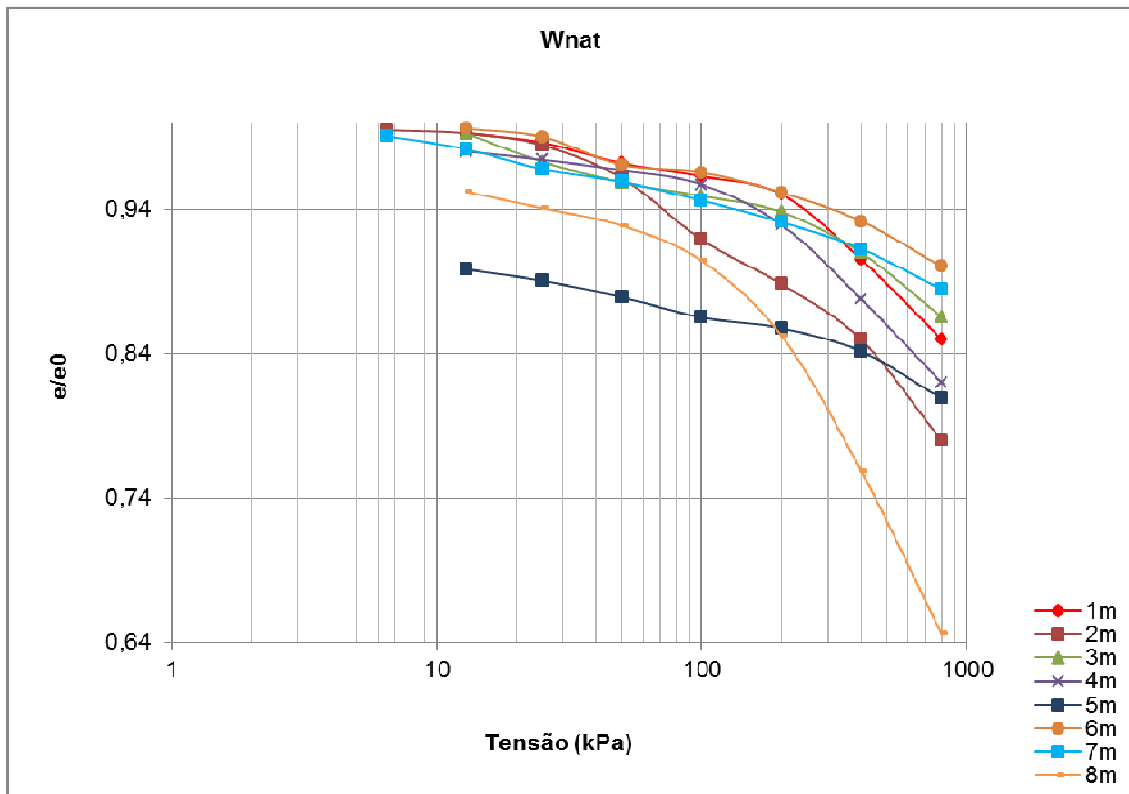
Figura 5.13 Curvas de Compressão edométrica normalizada do solo.
