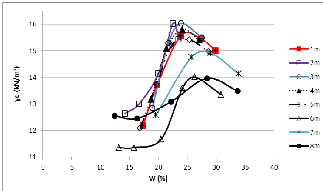
Figura 5.19 Curvas encontradas no ensaio de compactação na energia normal
