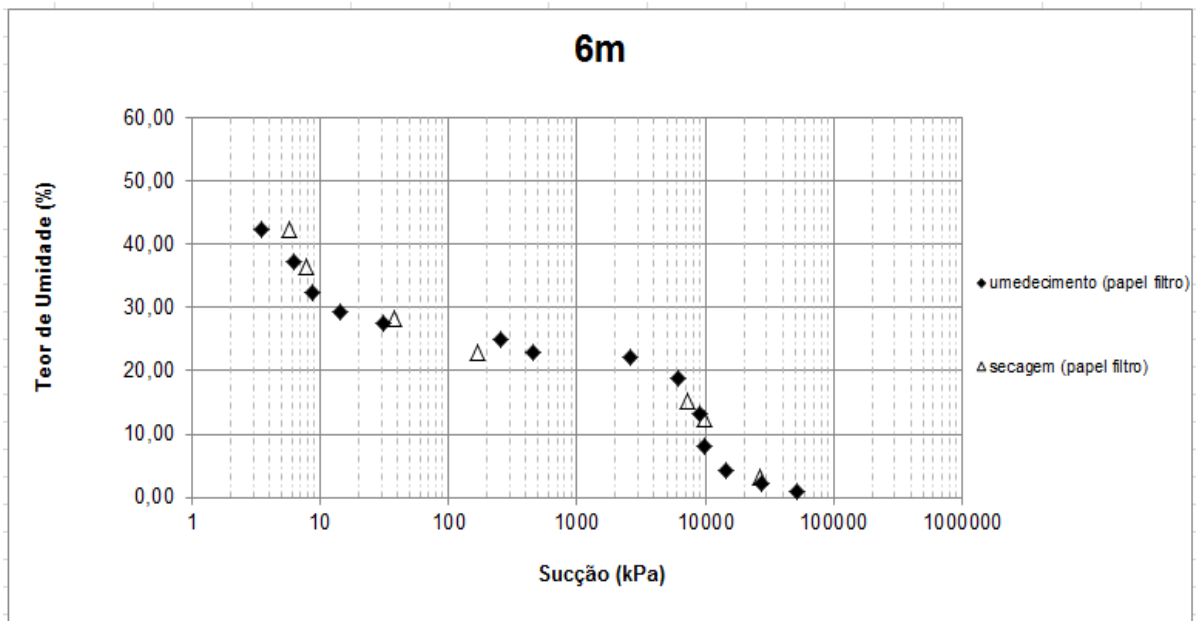
Figura 5.26 Curvas de retenção: teor de umidade gravimétrico vs sucção matricial -6,0m (papel filtro).
