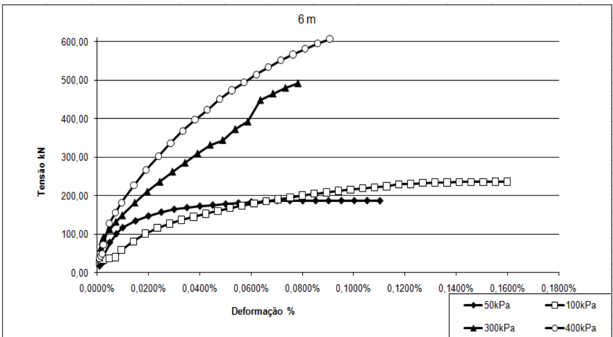
Figura I6- Comportamento tensão deformação para o sexto metro.
