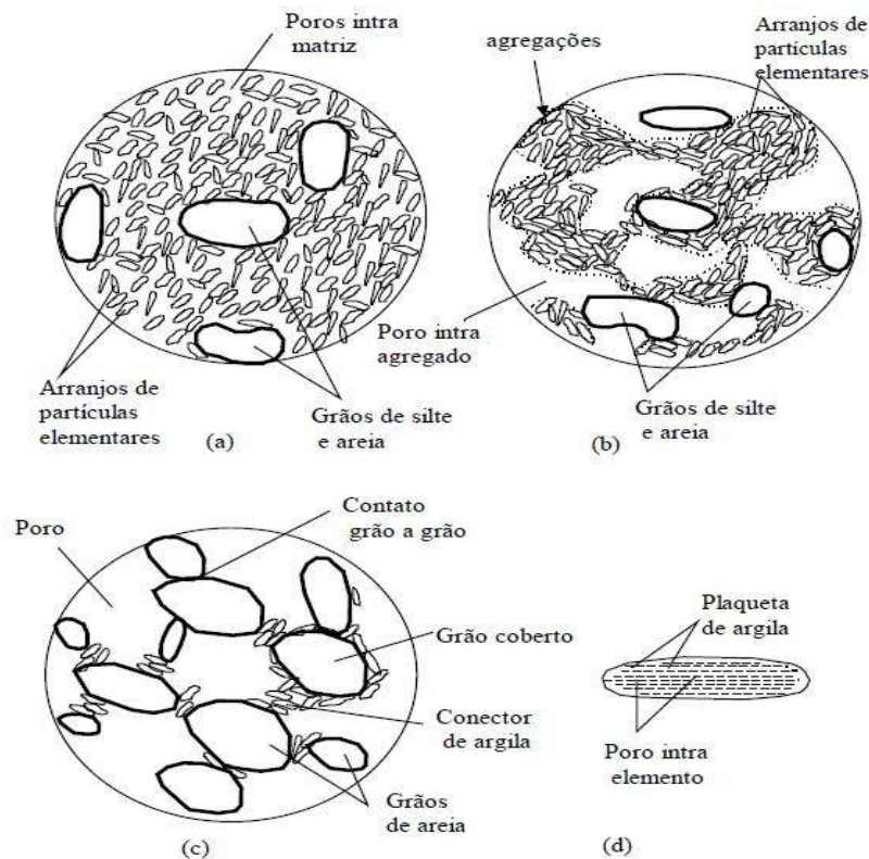
Figura 2.15. Arranjos microestruturais dos solos colapsíveis (Alonso et al, 1987). (a) Matriz de argila, (b) Microestrutura de argila constituída por agregações de arranjos elementares, (c) Matriz de silte e areia ligados por conectores de argila, (d) Arranjo elementar de argila na configuração paralela.
