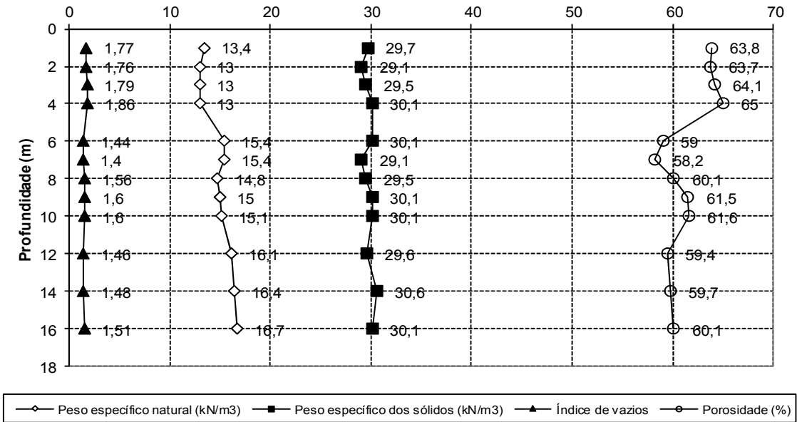
Figura 6.5 Valores de índices físicos obtidos por meio de ensaios laboratoriais e correlações do campo experimental da FEAGRI.
