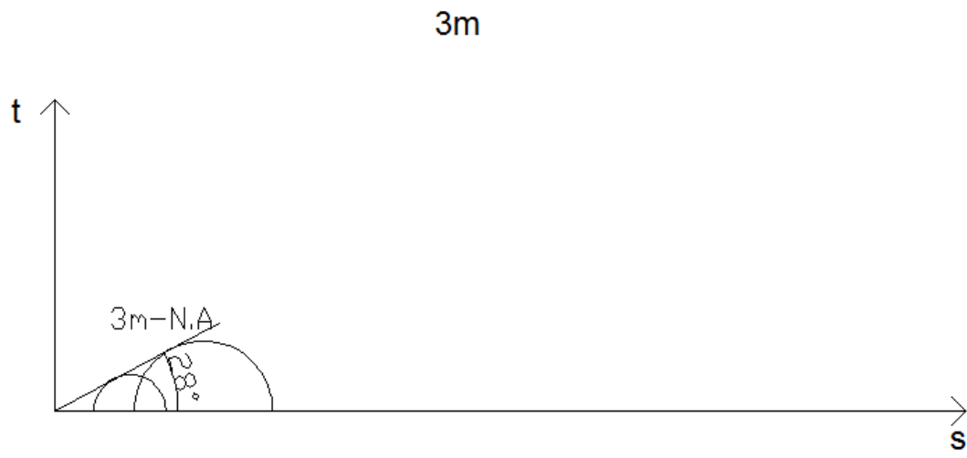
Figura II3- Envoltórias de resistência totais para o terceiro metro.
