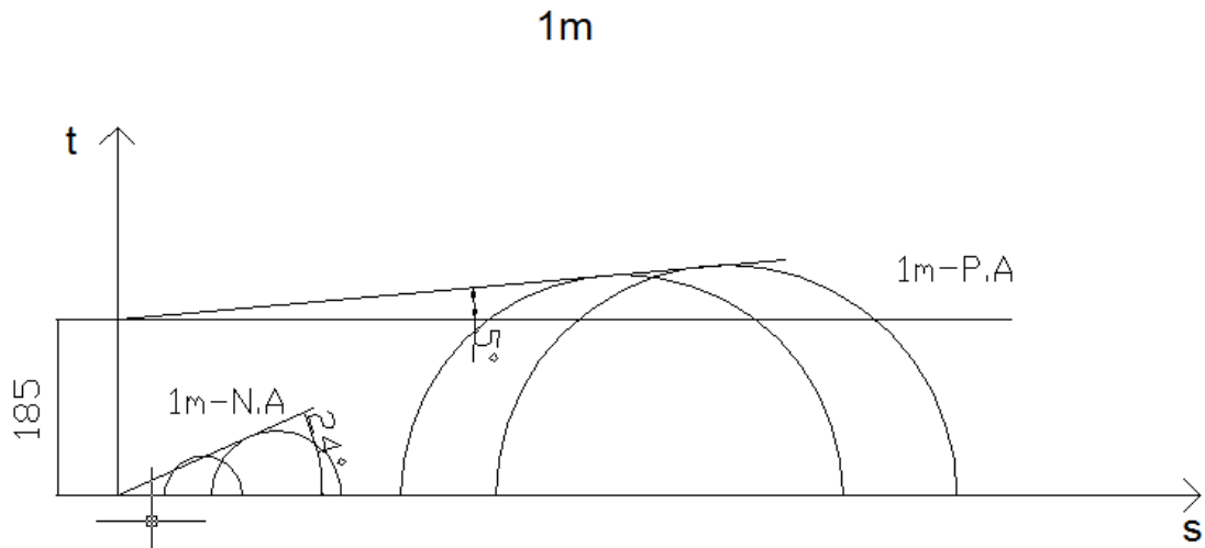
Figura II1- Envoltórias de resistência totais para o primeiro metro.
