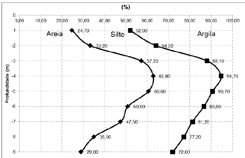
Figura 6.2 Variações das frações granulométricas do perfil com a profundidade do campo experimental da FEC
