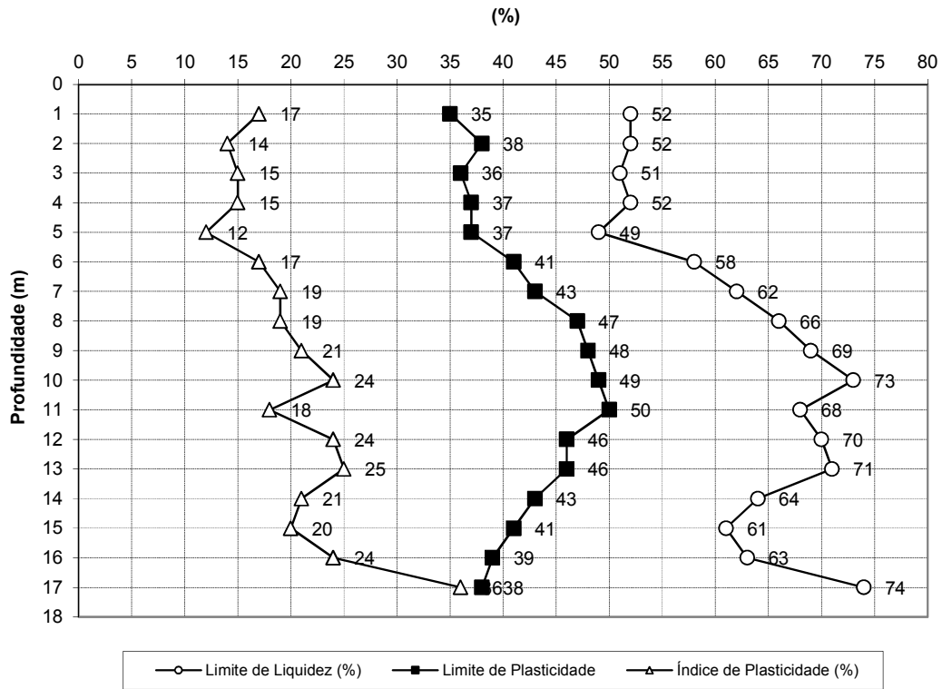
Figura 6.3. Variações dos limites de Atterberg em função da profundidade do campo experimental da FEAGRI
