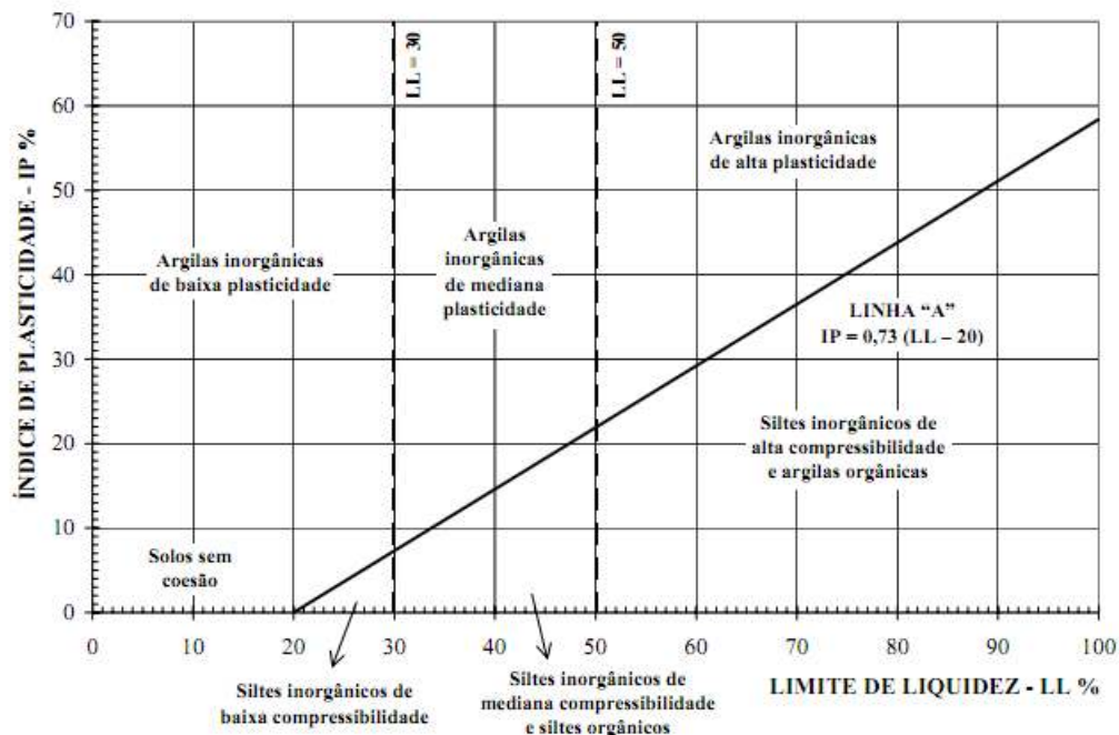
Figura 5.6 Classificação unificada proposta por Casagrande.
