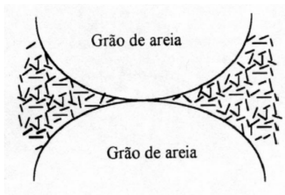
Figura 2.12. Arranjo estrutural devido a vínculos de argila resultantes do processo de lixiviação (Dudley, 1970).
