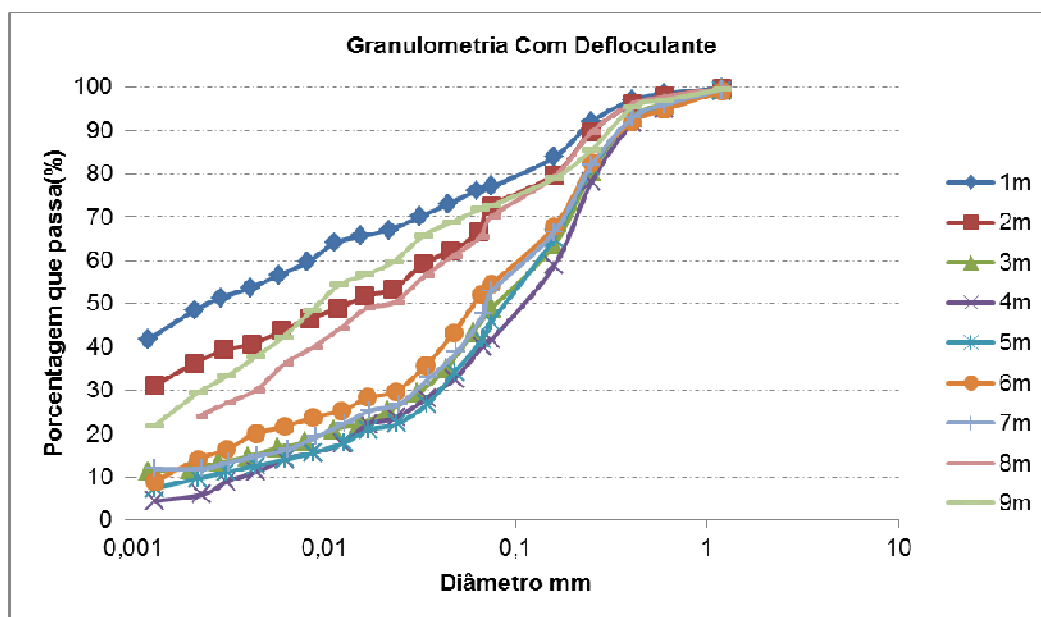
Figura 5.1. Curvas Granulométricas obtidas com o uso de defloculante.
