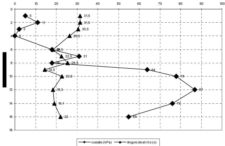
Figura 6.7. Parâmetros de resistência (tensões totais) obtidos em ensaios triaxiais (CU) do campo experimental da FEAGRI.
