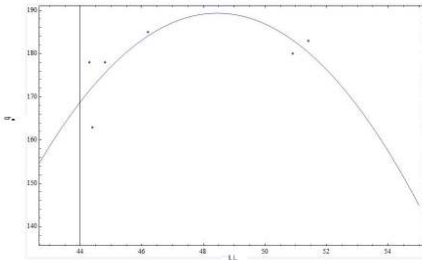
Figura 7.10 Modelo parabólico para correlação \sigma_a = f(LL)
