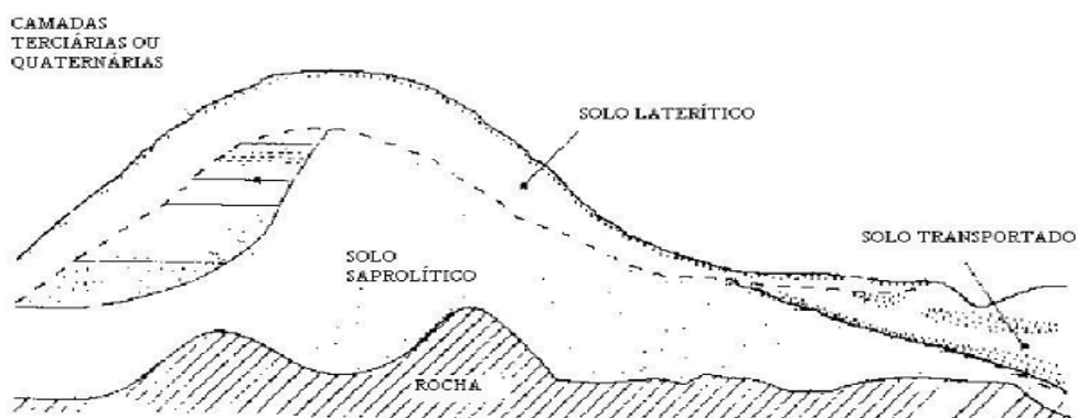
Figura 2.2. Perfil esquemático do subsolo em região de clima tropical (Nogami & Villibor, 1996).
