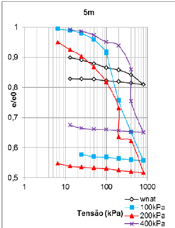
Figura 5.9 Efeito da inundação do solo em diferentes tensões para a profundidade 5m e 6 m.
