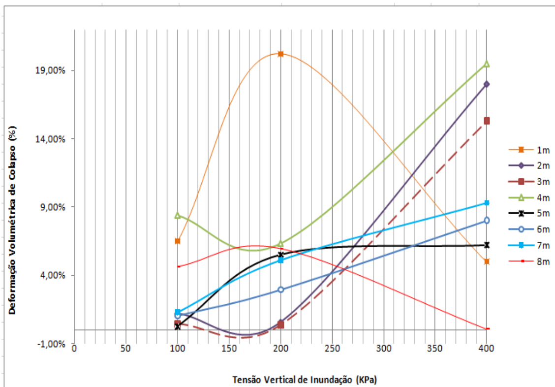
Figura 5.11 Variações dos coeficientes de colapso estruturais.
