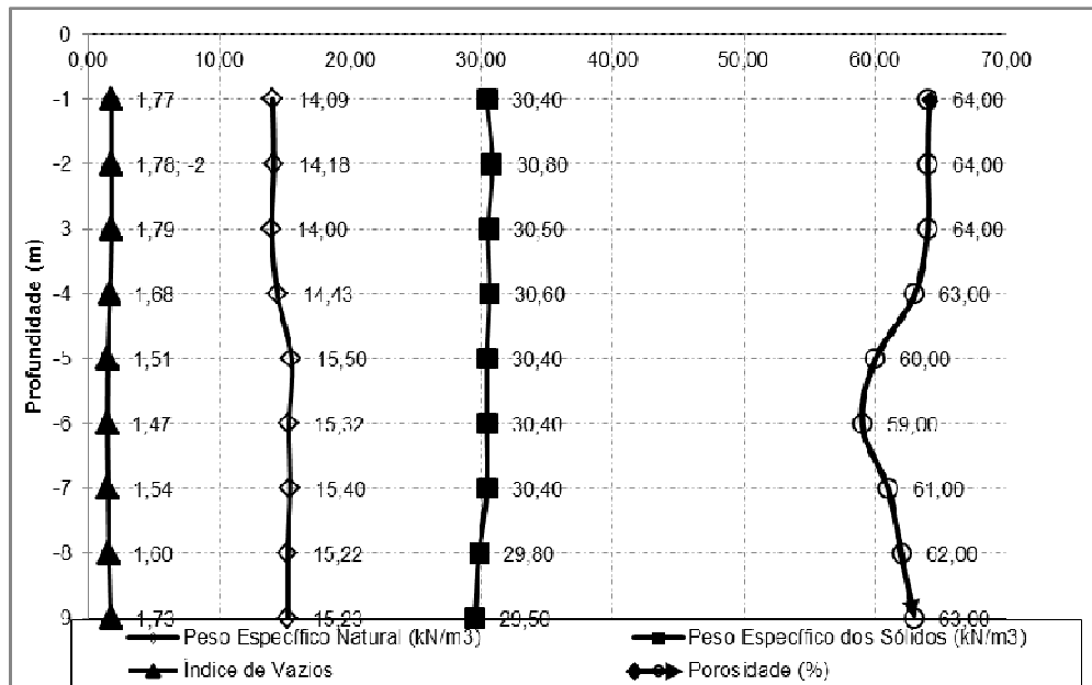
Figura 6.6. Valores de índices físicos obtidos por meio de ensaios laboratoriais e correlações do campo experimental da FEC
