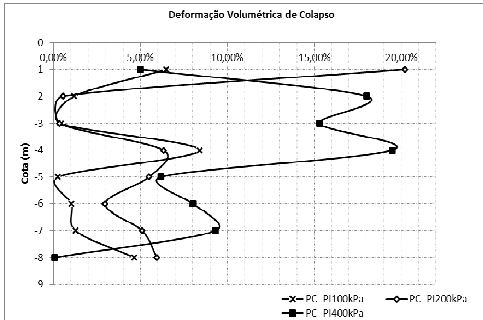
Figura 5.12 Variações dos coeficientes de colapso estruturais ao longo da profundidade.
