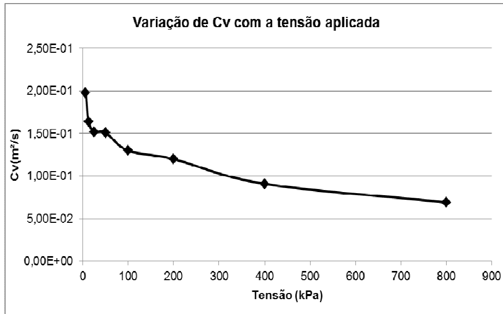
Figura 5.15. Variação de C_v com a tensão aplicada.
