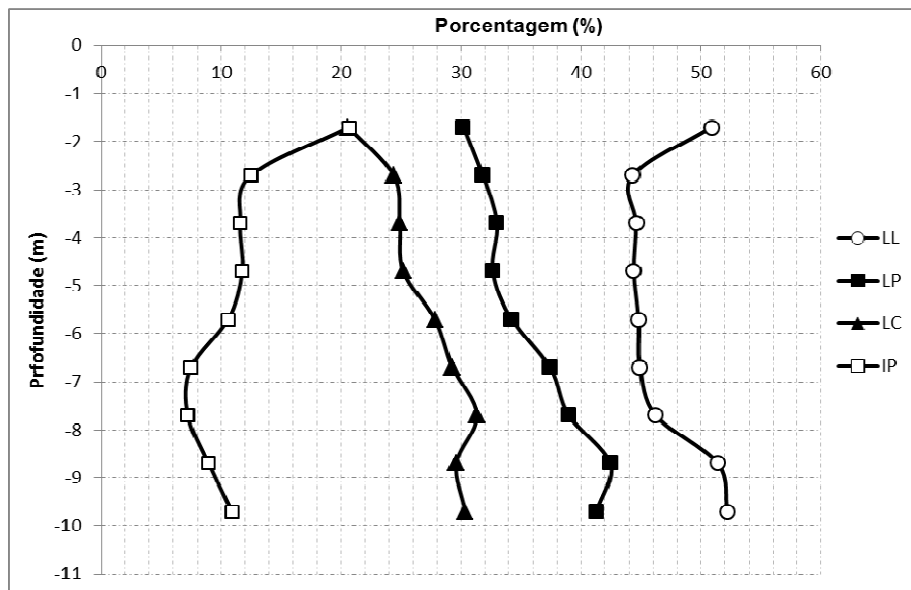
Figura 5.5 Valores de LL, LP, LC e IP ao longo do perfil estudado.
