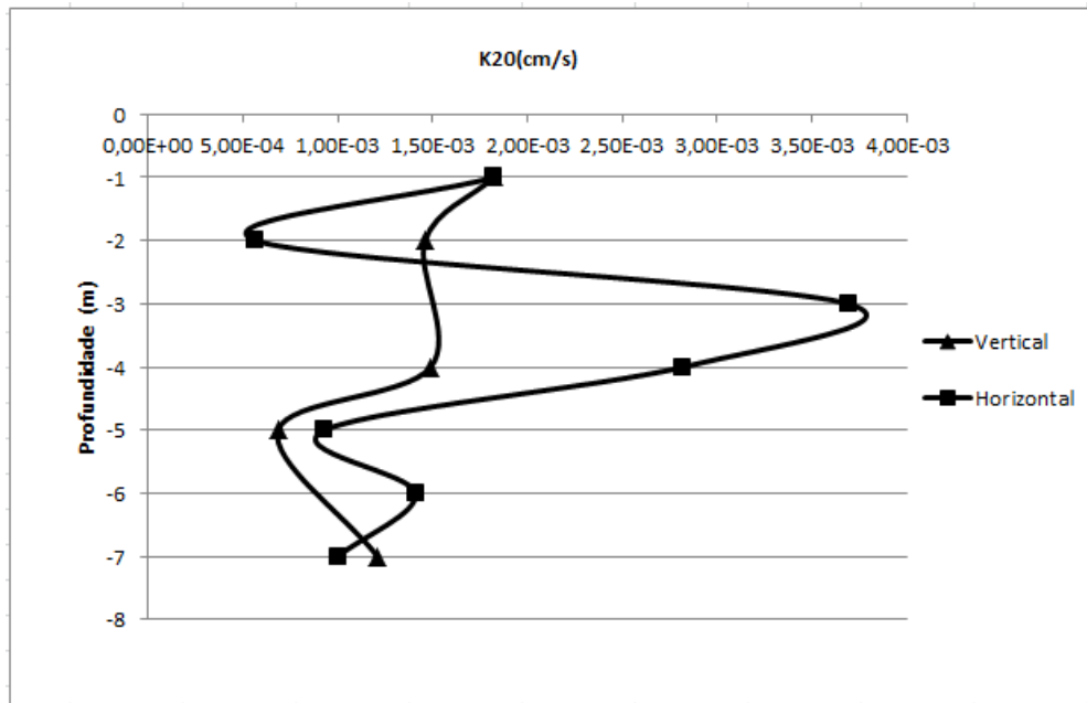
Figura 5.18. Condutividades hidráulicas vertical e horizontal vs profundidade.
