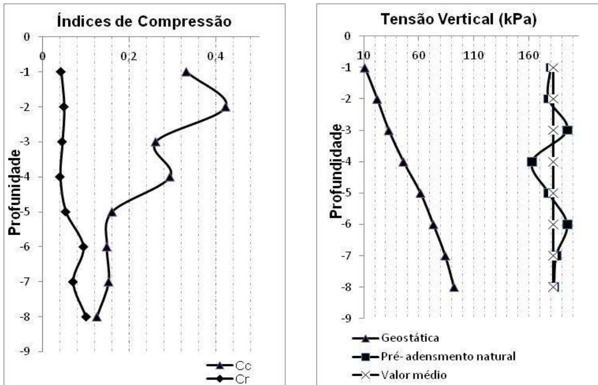
a) Índices de compressão e b) Tensões geostática e pré-adensamento
