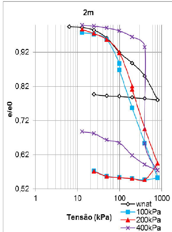
Figura 5.7 Efeito da inundação do solo em diferentes tensões para profundidade 1m e 2m.
