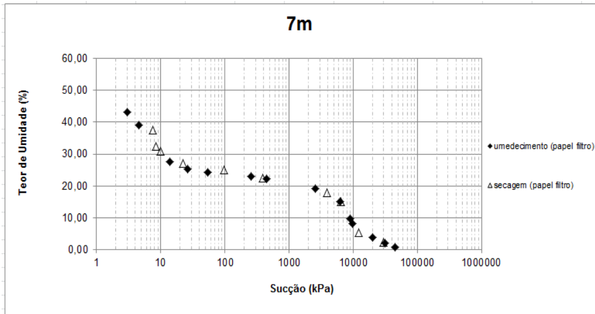
Figura 5.27 Curvas de retenção: teor de umidade gravimétrico vs sucção matricial -7,0m (papel filtro).
